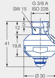
Kompakte Ausführung Außengewinde
